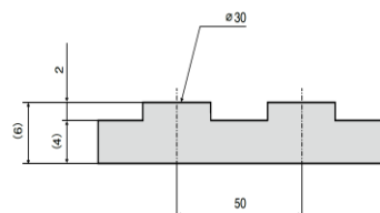
コイン形状参考断面図
