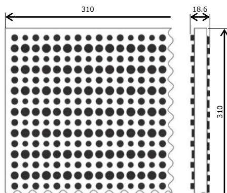
標準寸法図 定尺は310×310mmですが、設置条件に応じて自由にカットしたり、並べて使用できます。
